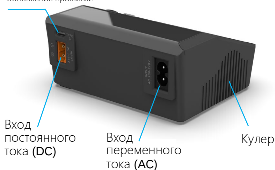
Вид сзади
